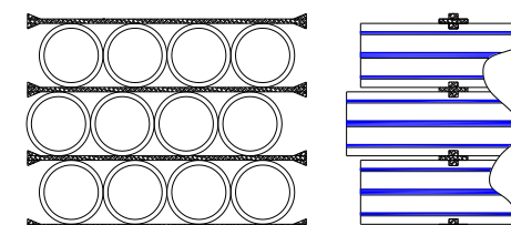
Stoccaggio ed impilaggio dei tubi sfusi Stacking & stacking of bulk pipes
