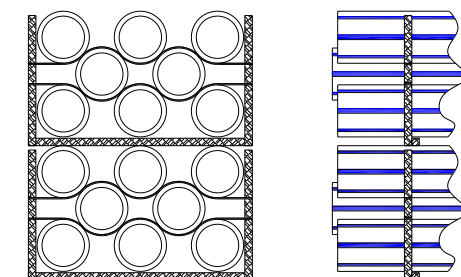
Stoccaggio ed impilaggio dei tubi in bancali Stacking & stacking of pipes in frames
